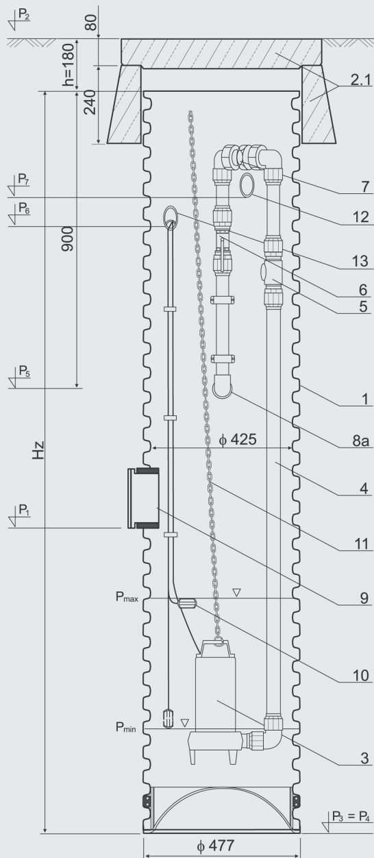
Rysunek złożeniowy minipompowni 425
