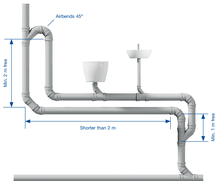
Fig. 24: Bypass pipe conforming to DIN 1986-100.
