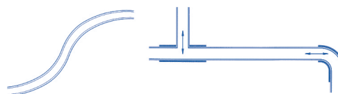
Figure 7 Absorption de l'expansion en cas de canalisation pourvue d'un fourreau ou d'une isolation
