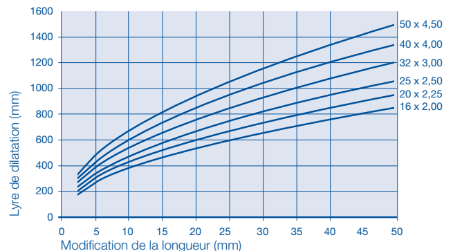
Figure 2 Calcul de la longueur des lyres de dilatation Wavin Tigris
