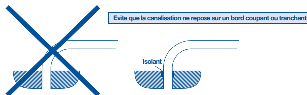
Figure 6 Protection des conduites Wavin Tigris émergeant d'un plancher ou d'une paroi
