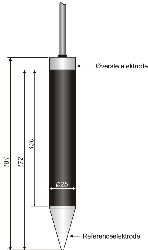
Figur 5. Måltegning af OMS-sensor
