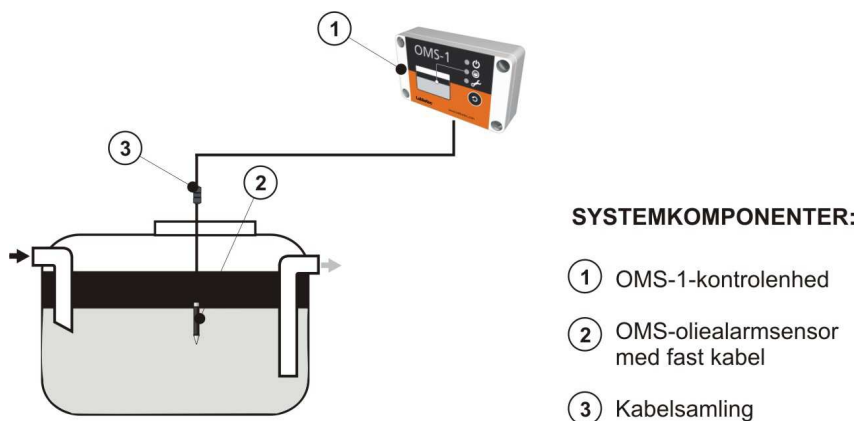
Figur 1. Overvågning af benzin- og olieudskiller med OMS-1-alarmenhed
