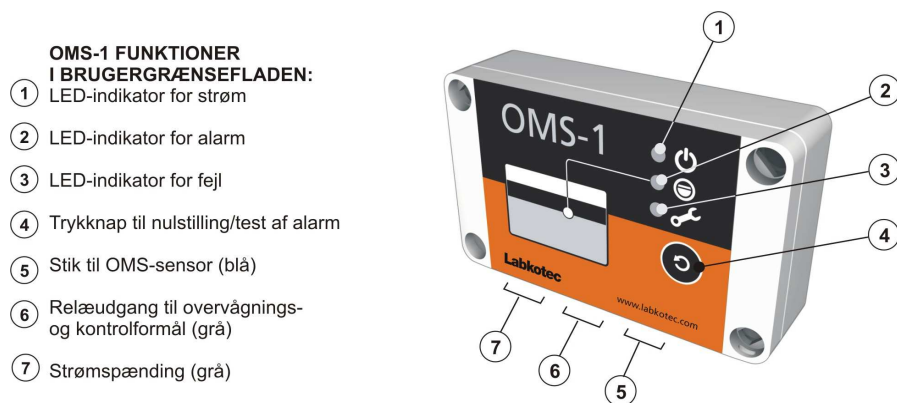
Figur 2. OMS-1-kontrolenhed – funktioner
