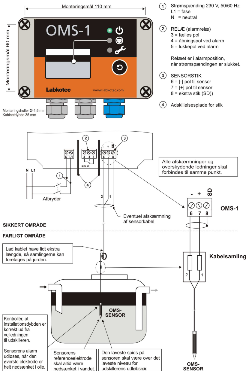
Figur 3. Installation af OMS-1-alarmenheden.
