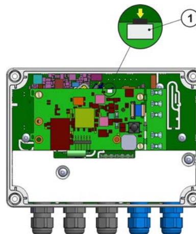
Figur 15. Sensoridentifikationsknap.
