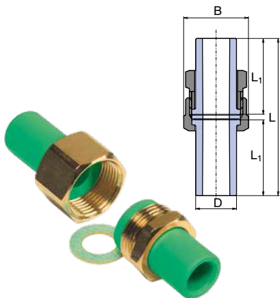
带螺母联轴节
