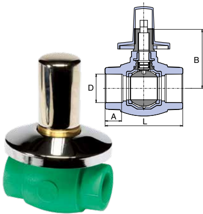
带镀铬盖的豪华直型球阀
