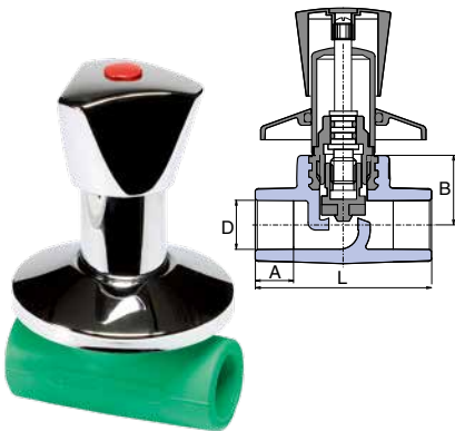
带镀铬盖的豪华款直型截止阀
