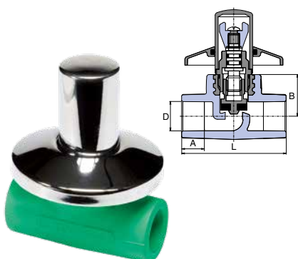
带镀铬盖的豪华款直型球阀
