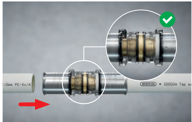
Mit dem 360° Sichtfenster lässt sich visuell prüfen, ob ein Rohr korrekt eingeführt wurde
