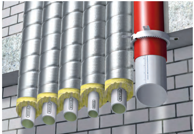
Brandschutz mit BM-R90 im Null Abstand
