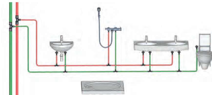
Traditionelles Verteilsystem, die sog. T-Stück Installation
