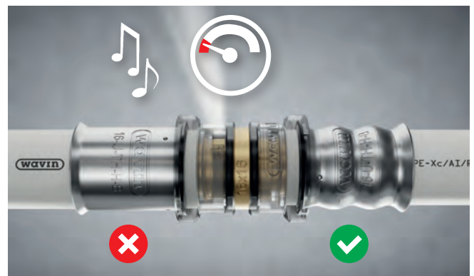
Akustisches Leckage-Signal bei Druckprüfung mit Luft
