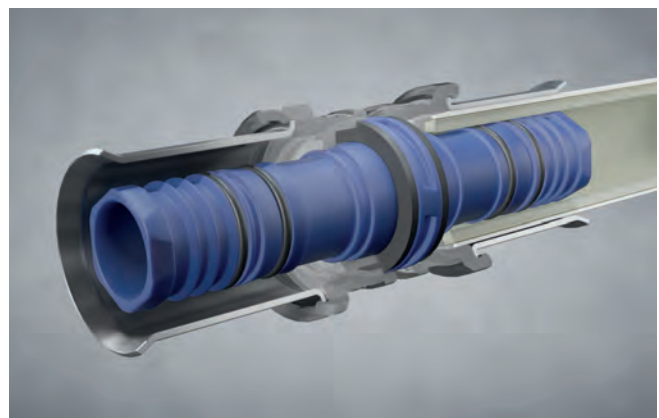
Einstecken der Rohrleitung ohne Kalibrierung dank geringer Einsteckkräfte
