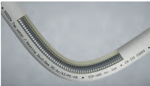
Biegen des Rohrs mit einer Biegefeder
