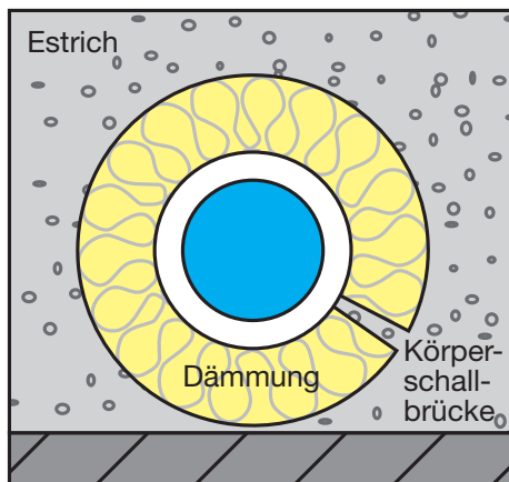
Übertragung von Körperschall durch defekte Rohrdämmung
