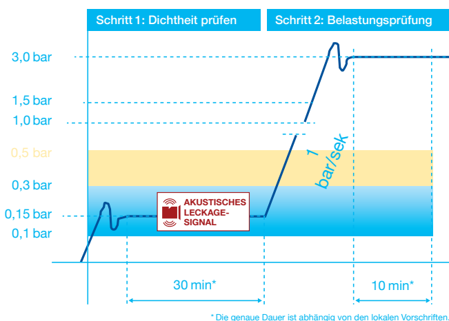
Protokoll Druckprüfung bei Prüfung mit Luft
