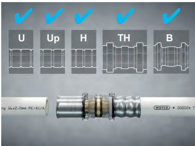
Fünf Konturen – Verpressung mit den gängigsten Presskonturen möglich
