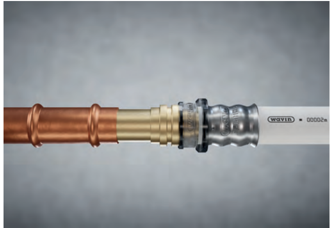
Übergang auf Kupfer, C-Stahl und Edelstahl mit Tigris M5
