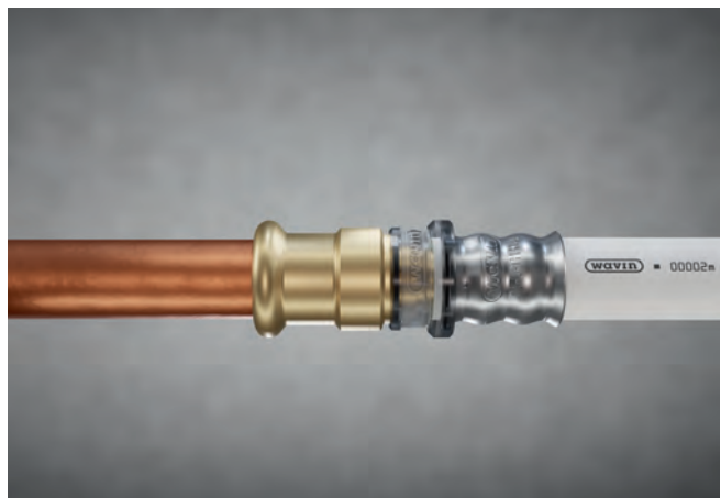
Pressübergang auf Kupfer, C-Stahl und Edelstahl mit Tigris M5
