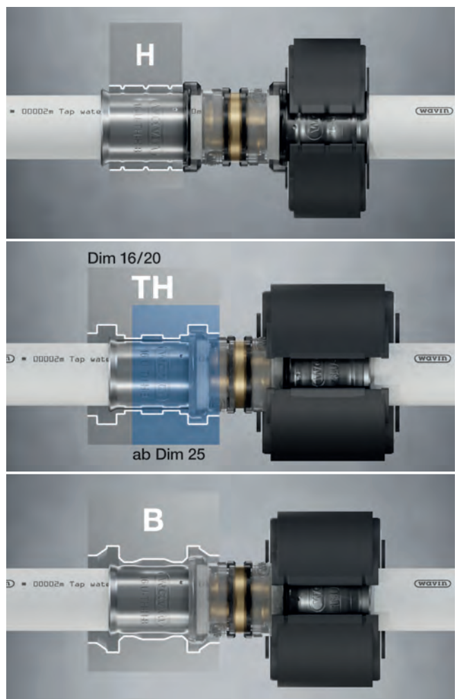
Freigegebene Presskonturen für Tigris K5/M5
