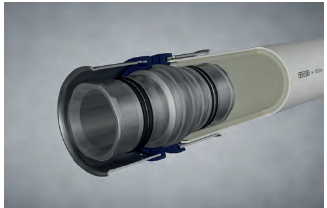
Geringe Einsteckkräfte durch den patentierten Sechskant-Querschnitt
