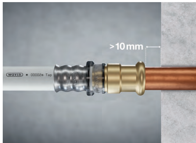
Mindestabstand von Fitting zu Wand
