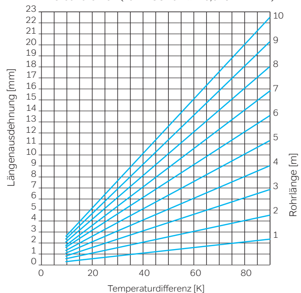
Thermisch bedingte Längenausdehnung von Wavin Mehrschicht-Verbundrohren (auf Basis von \alpha = 0,025 \text{ mm/m}\cdot\text{K} )
