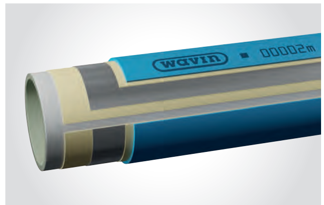
Mehrschicht-Verbundrohr für Niedertemperatur-, Heizkörperanbindung und Fußbodenheizungsinstallation
