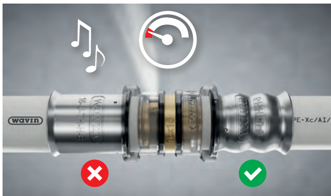
Akustisches Leakage-Signal – anhand eines lauten Pfeiftons, der durch die austretende Luft verursacht wird, lassen sich unverpresste Fittings schnell identifizieren
