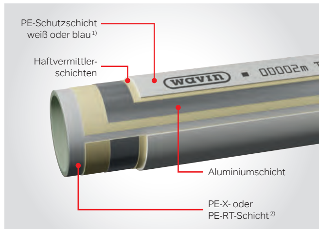
Mehrschicht-Verbundrohr-Aufbau
