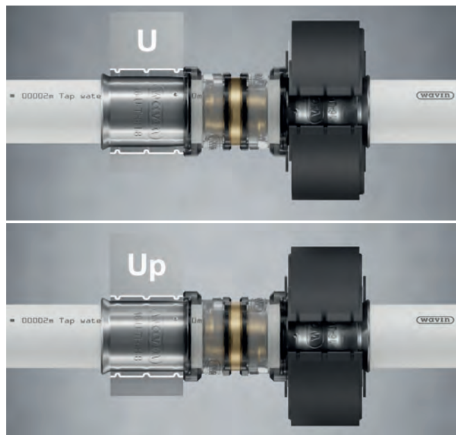
Freigegebene Presskonturen für Tigris K5/M5
