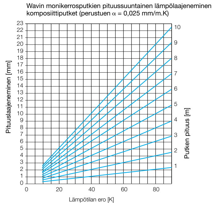
Kuva 36: Pituussuuntainen lämpölaajeneminen.
