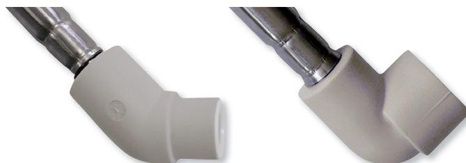
Připojení k radiátoru – koleno 45° a 90°
