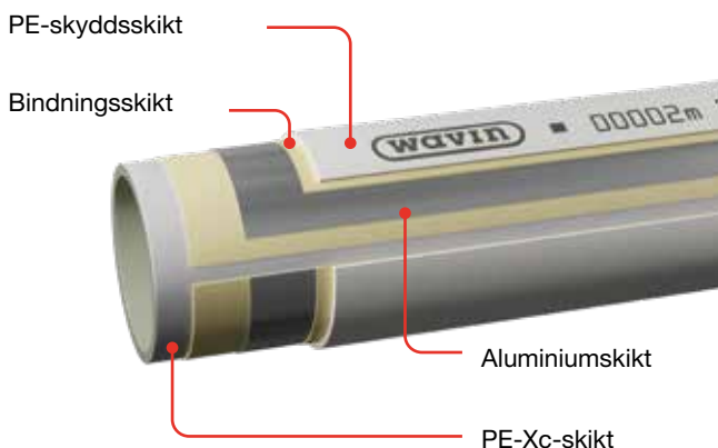
Fig. 1: Struktur, Wavin flerskiktssystem.
