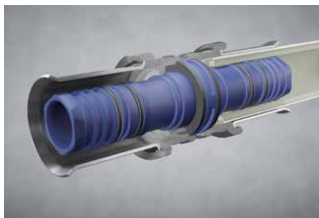
Fig. 10: EASYFIT rörsättning utan kalibrering.
