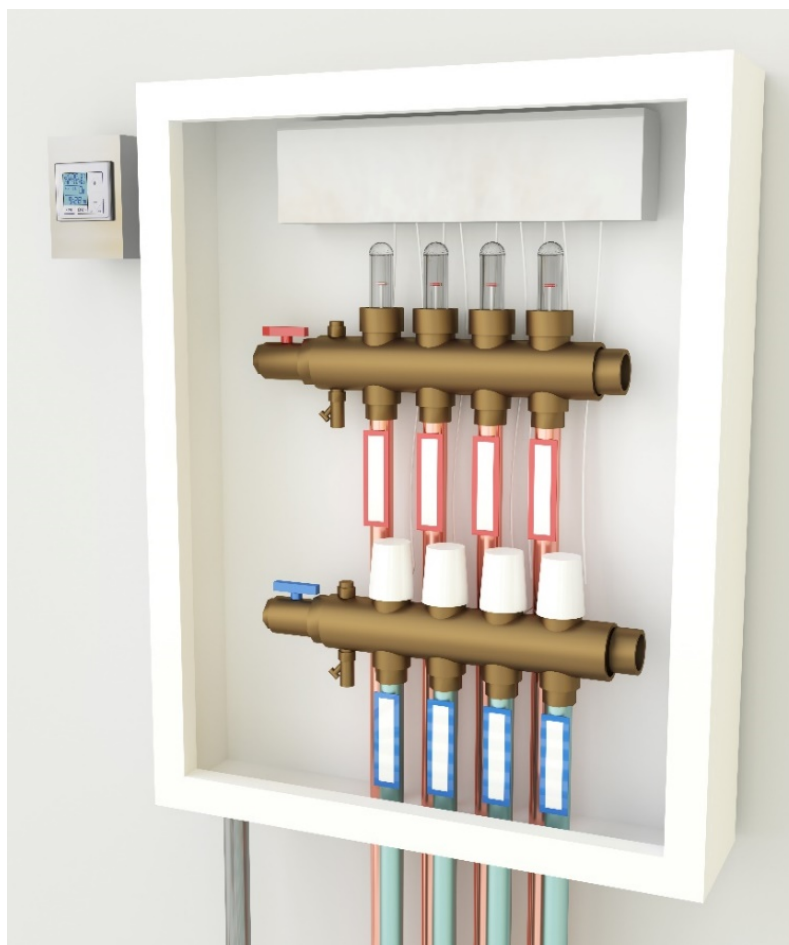
Figur 3 – Illustrasjon av fordelerskap med overløp som inneholder fordelerstokk, aktuatorer og kontrollenhet.
