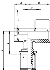
Wavin M5 – Nástěnné koleno 90° – vnitřní závit prodloužený
