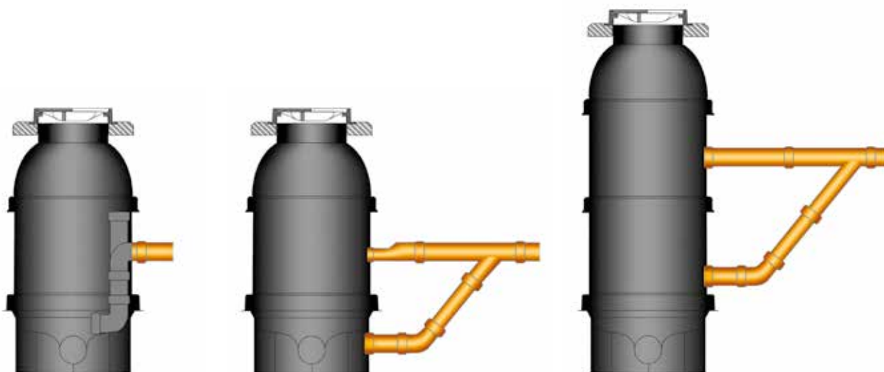
Przykładowe rozwiązanie kaskad przy studzienkach włączonych
