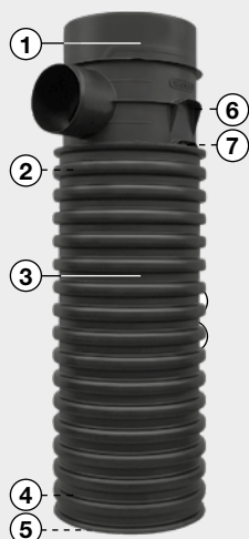
XL (100-200 dm 3 ) z elementów do trzonu D sr 450
