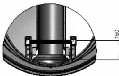
Usytuowanie szczelki drabinki w świetle otworu wlotowego stożka – widok z góry.
