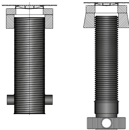
Rysunek 1. Przykładowe rozwiązania studzienek z kinetą przepływową wykonane z rur strukturalnych:
