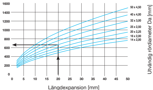
Fig.: Böjfogsklassificering Wavin flerskiktströr.
