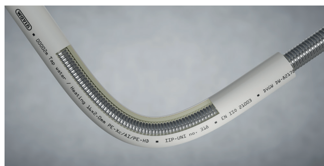
Bockning av röret med enbockningsfjäder.
