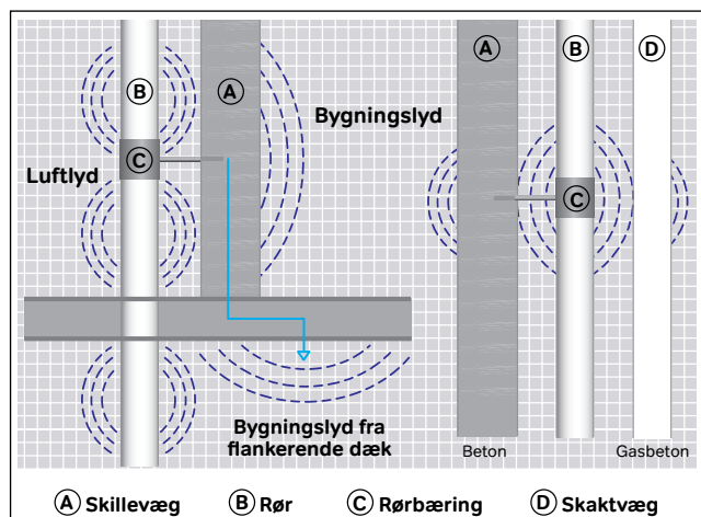
Eksempel på lydudstråling fra flankerende bygningskonstruktioner.
