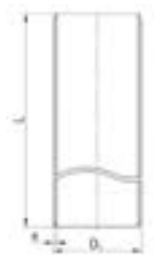
KG aknafalcső DN400 SN2
