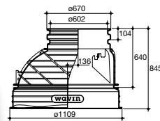
Tegra 1000 NG szűkítő
