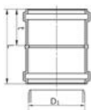
Acaro PP SN 12 kettős karmantyú*
