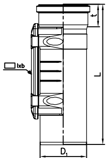
KGRE tisztítónyílás
