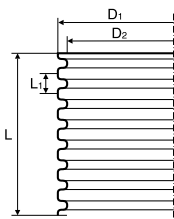
Aknafalcső DN600 – SN \geq 4 \text{ kN/m}^2
