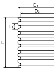
Aknafalcső DN600 – 2 \leq SN < 4 \text{ kN/m}^2
