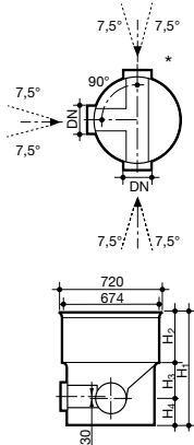
Tegra 600 aknafenek – oldalbekötő
