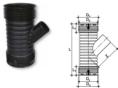
X-Stream PP ágidom 45° – KG átmeneti idom*
