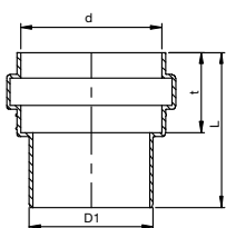
GREEN CONNECT 2000 PP átmeneti idom kőagyag csőhöz – csővégre*
