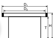
Tegra 800 teleszkópcső
