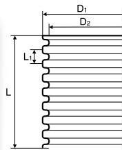
Aknafalcső DN600 – 2 \leq SN < 4 \text{ kN/m}^2
