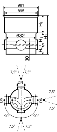
Tegra 800 aknafenek – elágazó 90°
