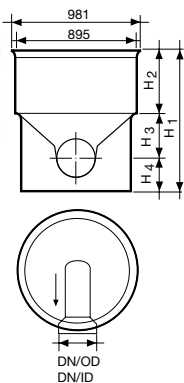
Tegra 800 aknafenek – végakna
