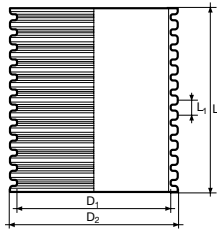
Tegra 1000 NG aknafalcső
