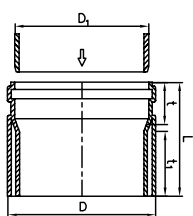
KGUSM átmeneti idom kőagyag csőhöz
