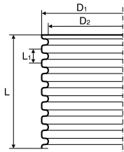
Aknafalcső DN600 – SN \geq 4 \text{ kN/m}^2
