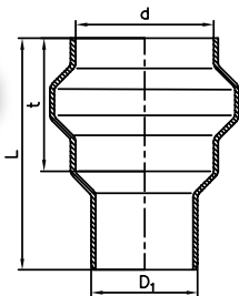
KGUS átmeneti idom kőagyag csőhöz
