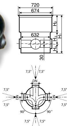
Tegra 600 aknafenek – elágazó 90°
