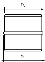
Bordás aknafalcső toldóidom – 2 db gumigyűrűvel D315
