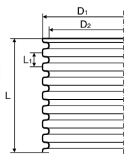
Aknafalcső DN315 – SN ≥ 4 kN/m 2
