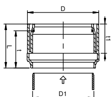
GREEN CONNECT 2000 PP átmeneti idom kőagyag csőhöz – tokba*
