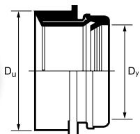
Aknafal-csatlakozócsok
