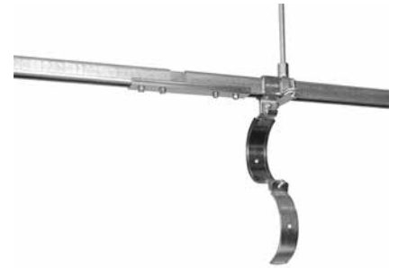
Figura 72. Nel bracciale scorrevole nessuno inserto deve essere utilizzato.
