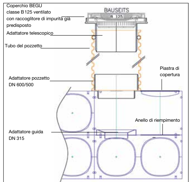
Sovrastruttura del pozzetto a due strati Q-bic
