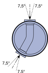
Tipo I/flujo di base 30° Angolo di regolazione nell'intervallo di 15° - 45°
