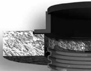
Chiusino su anello di sostegno in CLS
