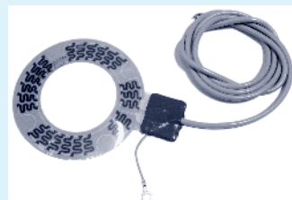
Elemento riscaldante elettrico antighiaccio 230 V/18 W ID 140 mm
