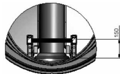
Posizione dei gradini rispetto all'accesso dal cono – vista dall'alto
