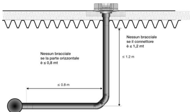
Figura 79. Nessun bracciale verticale se il tubo di scarico verticale \leq 1,2 metri. Nessun bracciale di supporto orizzontale se il tubo di scarico orizzontale \leq 0,8 metri.
