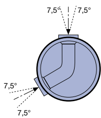
Tipo I/flujo di base 60° Angolo di regolazione nell'intervallo di 45° - 75°
