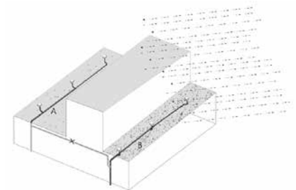
Figura 12. Soluzione preferita per diverse condizioni di copertura.
