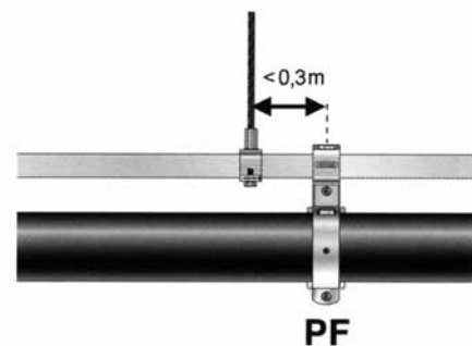
Figura 78. Punto Fisso max 0.3 mt dall'elemento di sospensione.
