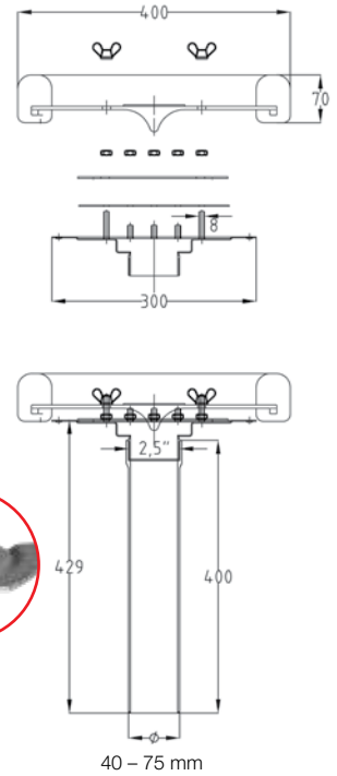
Capacità di scarico QS-M-75-400, per coperture in membrana
