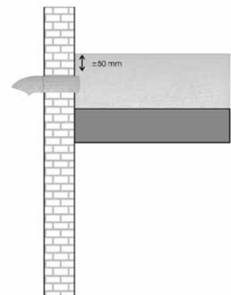
Figura 27. Calcolo di un troppopieno di emergenza rettangolare
