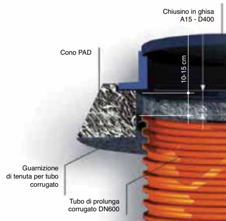
COPERTURA CON CONO PAD
