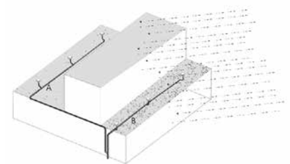
Figura 13. Collegamento sopra il livello del solaio.
