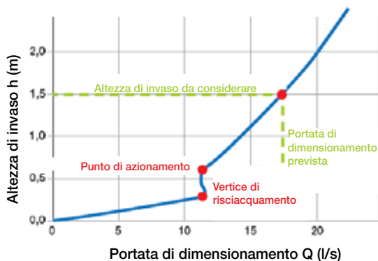
Organo di regolazione della portata Vortex Modello FC 12 con
