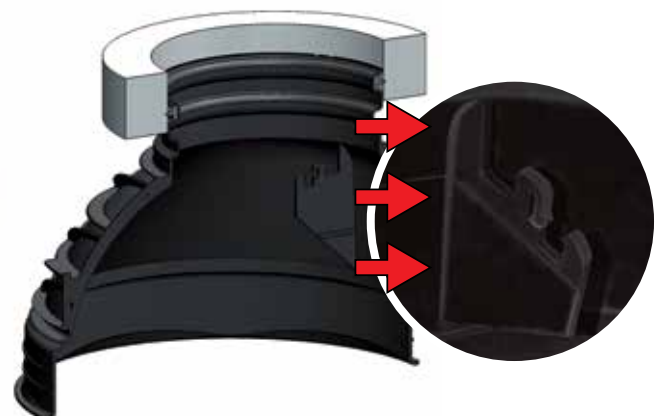
Foto 5. Dettaglio - supporto superiore della scala - staffa installata nel cono.
