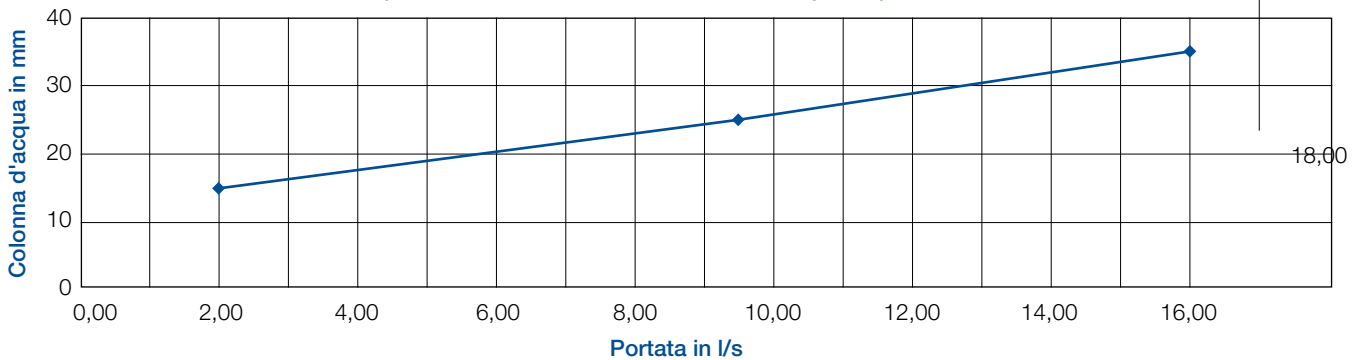
Capacità di scarico ricettore QS-M-75-400, per coperture in bitume
