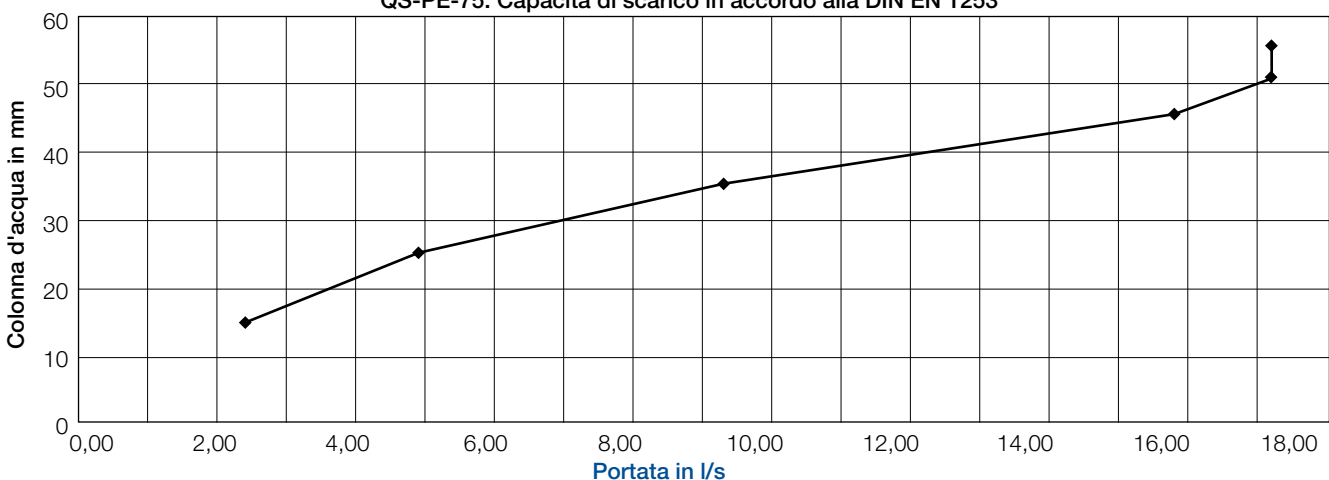
Prestazioni QS-PE-75 (in accordo alla DIN EN 1253)
