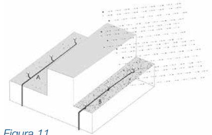
Figura 11. Le sollecitazioni del vento possono causare carichi diversi sulle diverse zone del tetto.
