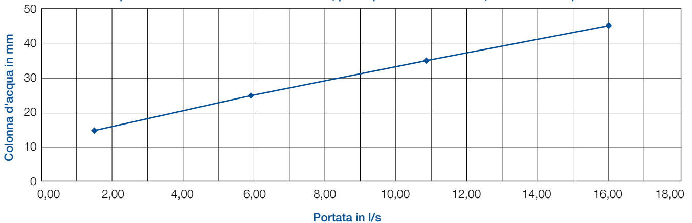
Prestazioni ricettore QS-M-75-260, per coperture in membrana (DIN EN 1253)
