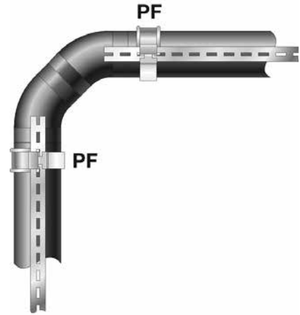
Figura 77. Collocazione dei bracciali a punto fisso prima e dopo una curva (vista dall'alto).
