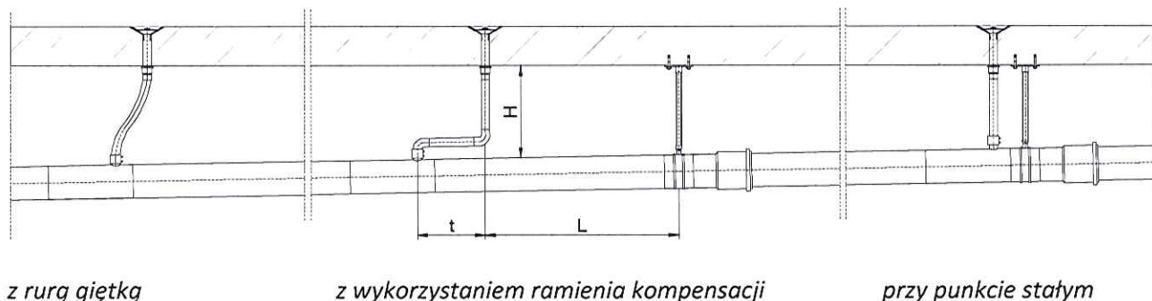
Rysunek Z2-2 - Metody przyłączania sączka do instalacji odwodnieniowej WAVIN
