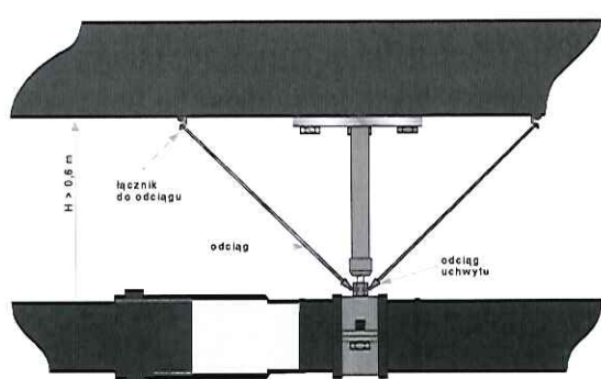
Rysunek Z2-3 - Przykład mocowania rury odwodnieniowej z wykorzystaniem odciągów: a) górnego, b) bocznego
