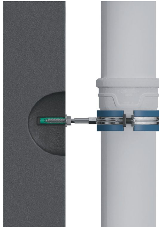
Zusätzliche Fallrohrsicherung mit Hilfe einer Festpunktauflage
