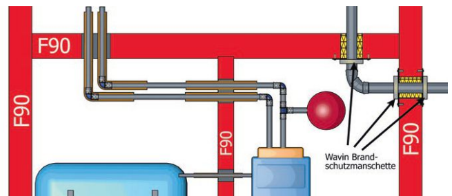
Abb. 26: Brennstofflagerräume und Heizraum getrennt mit: >5.000 Liter Heizöl oder > 15.000 kg Festbrennstoffe oder > 14 kg Flüssiggas.
