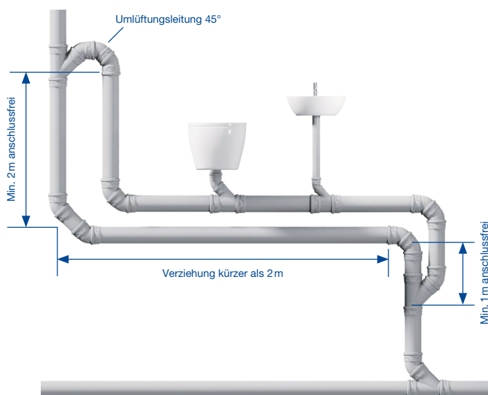
Abb. 9: Fallleitungsverziehung < 2m mit Umgehungsleitung und anschlussfreien Leitungsbereichen
