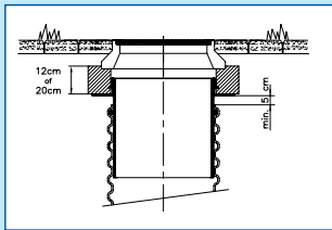
Put met betonafdekking, incl. telescoop
