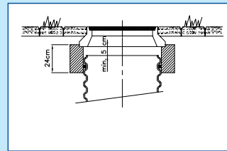
Put met betonafdekking, excl. telescoop
