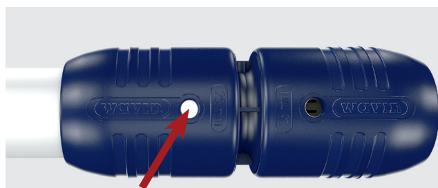
9. ábra: A kupakban található kémlelőnyíláson keresztül ellenőrizhető a cső ütközésig történő betolása
