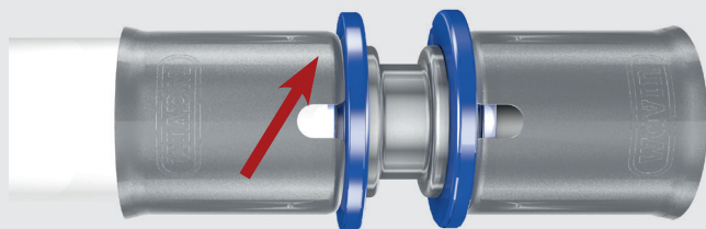
6. ábra: A rozsdamentes acél préshüvelyben található kémlelőnyíláson keresztül ellenőrizhető a cső ütközésig történő betolása
