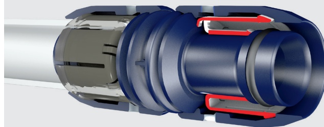
10. ábra: A Wavin smartFIX idomrendszer
