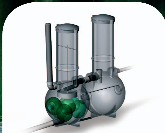
Labko® BioRami 500 0,5 m³ LVI-numero 3629 005
