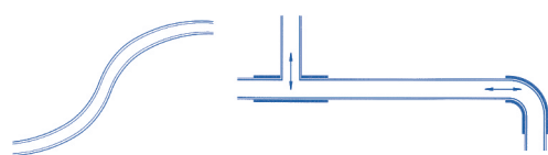
Afb. 7 Opvangen van expansie bij leiding met mantelbuis door royaal leggen en door isolatie
