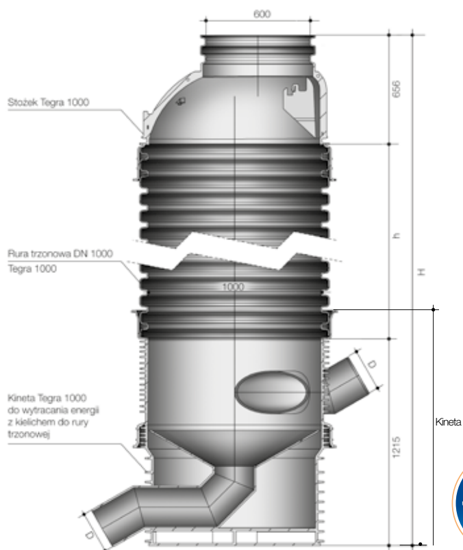
Charakter przepływu w studzience do wytracania energii
