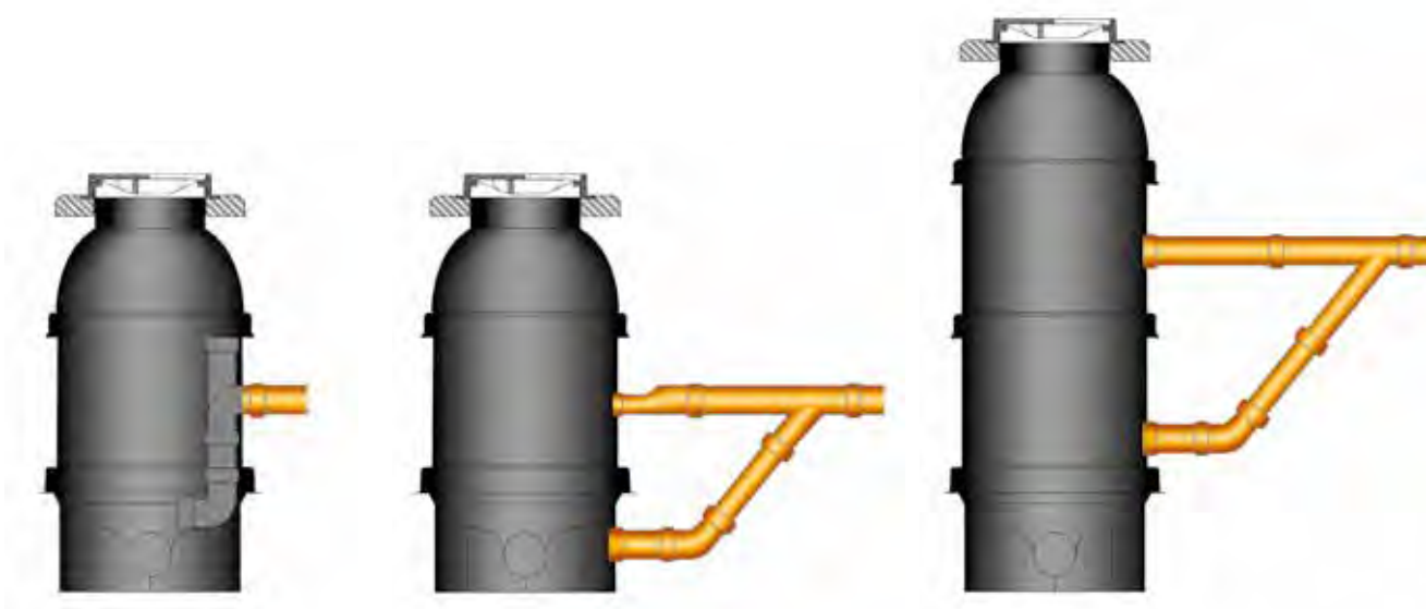
Przykładowe rozwiązanie kaskad przy studzienkach włączonych
