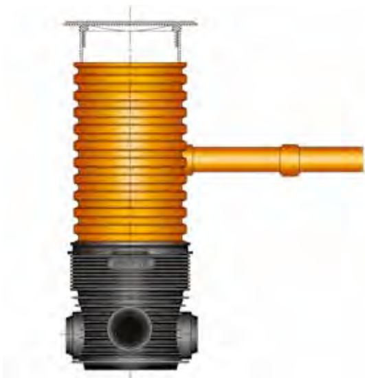
Przykładowe rozwiązania kaskad przy studzienkach niewłazowych
