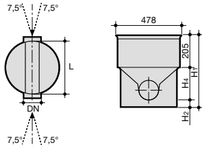
Kineta Tegra 425 do rur gładkościennych – króćce SW
