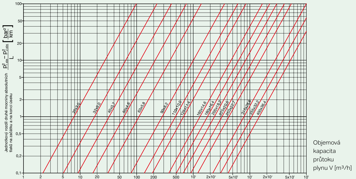
Nomogram PE 100 a PE 100 RC potrubí SDR 11 pro střední a vyšší tlaky plynu
