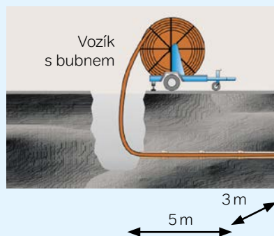
Startovací výkop během zatahování potrubí
