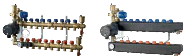
Wavin parallelshunt med- og uden isoleringsskåle
