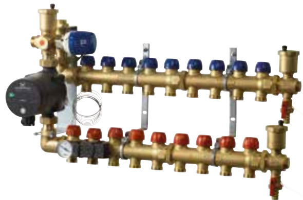
Parallellshunt sammen med fordelerrør og endestykkesett.
