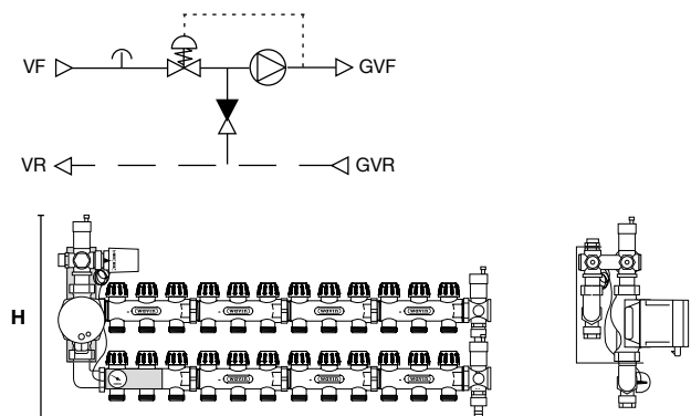
Parallellshunt sammen med fordelerrør og endestykkesett.
