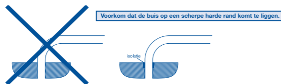
Afb. 6 Het beschermen van uit de wand of vloer komende leidingen
