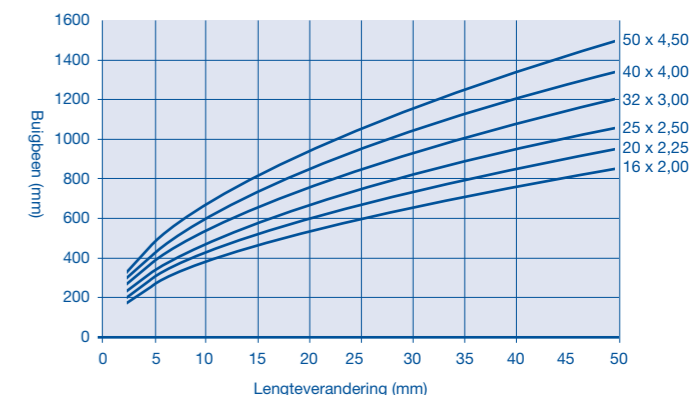
Afb. 2 Bepaling van de buigbeenlengte bij Wavin Tigris
