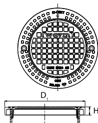
Litinný poklop A15 – do šachtové roury
