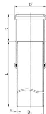
Acaro PP SN 16 – trubka s dvouhrdlou spojkou
