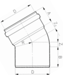
Solidwall PVC SN12 - Koleno 45°
