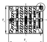
Litinná mříž D400 Ø 315 mm – do teleskopické roury
