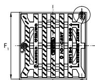
Litinná mříž D400 Ø 425 mm – do teleskopické roury
