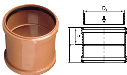
KG PVC-U - Spojka dvouhrdlá
