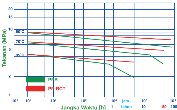
Diagram Garis Mekanisme Isotermal - PPRCT dan PPR
