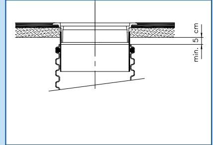
Put met drijvend deksel
