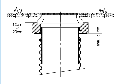
Put met betonafdekking, incl. telescoop
