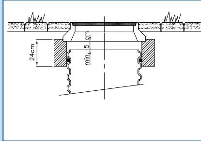
Put met betonafdekking, excl. telescoop
