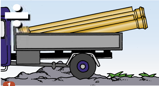
1 Transporter rør og fittings i fabriksemballagen. Sørg for, at rørene ikke beskadiges af skarpe kanter og genstande, hvis rørbundter skal deles.
