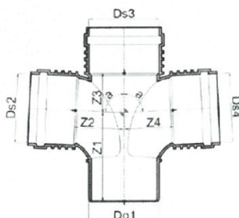
Rys. A7. Czwórniki proste systemu WAVIN SiTech+
