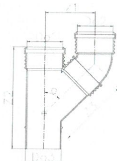
Rys. A5. Trójniki specjalne (shower branch) systemu WAVIN SiTech+
