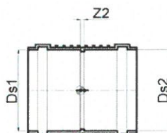
Rys. A13. Mufy z wydłużonym kielichem systemu WAVIN SiTech+
