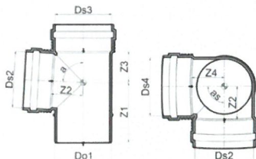
Rys. A8. Czwórniki radialne systemu WAVIN SiTech+
