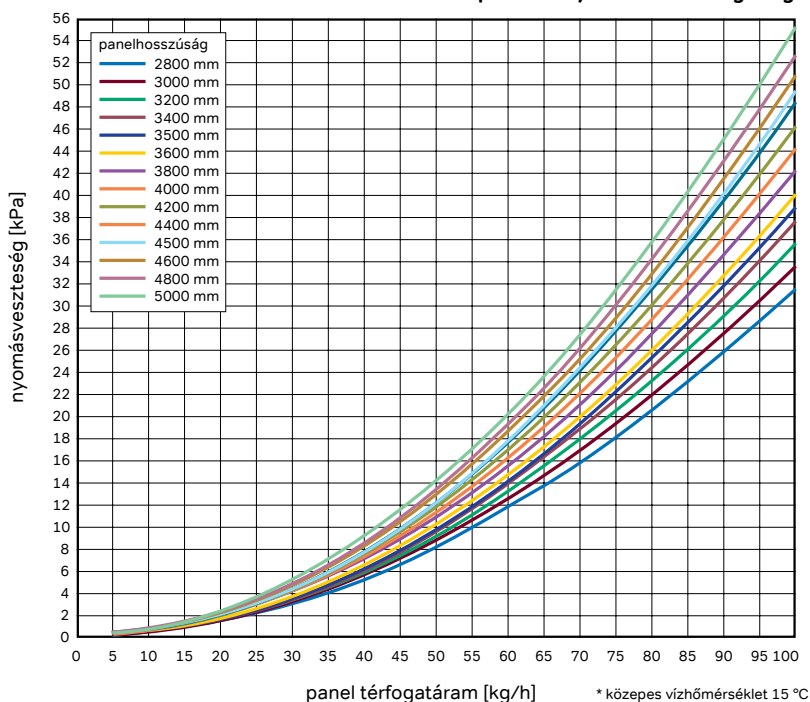
Wavin Comfia CD-4 felületfűtési -hűtési panelek nyomásvesztés diagramja*
