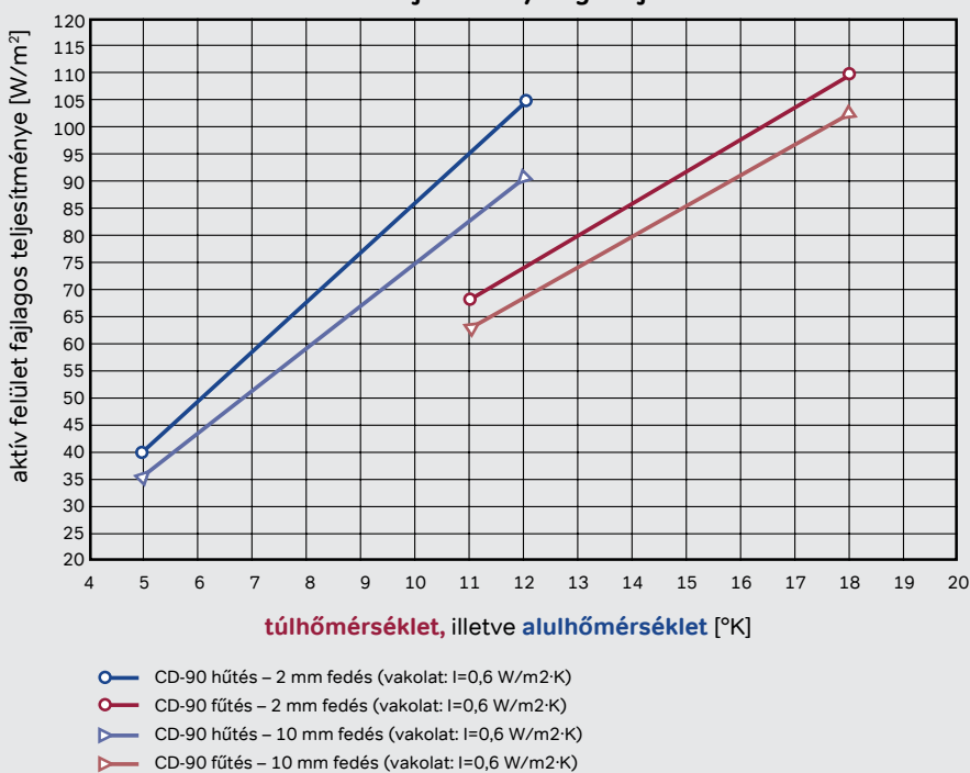
Wavin Comfia CW-90 felületfűtési -hűtési rendszer teljesítménydiagramja
