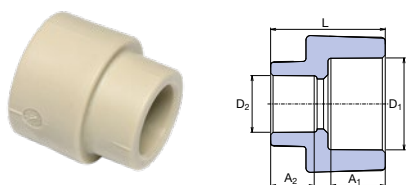
Redukce hrdlová
