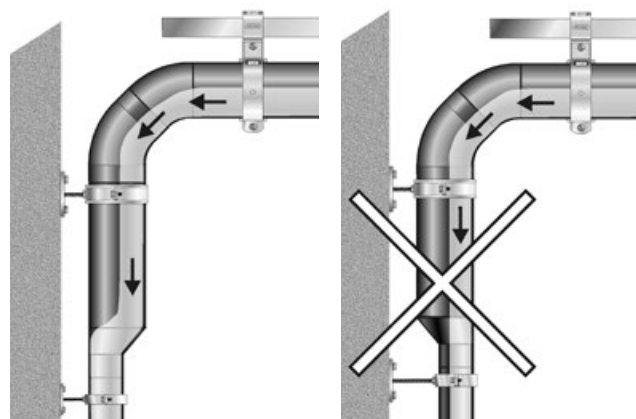
Umístění excentrických redukcí pro případ vertikálního potrubí
