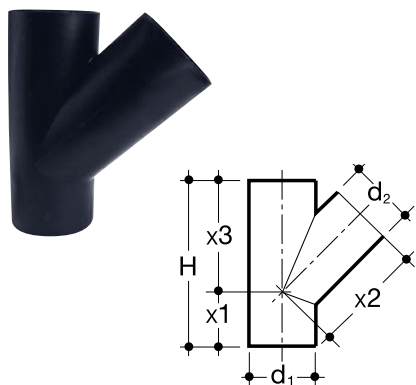
Odbočka 45° – SDR 33
