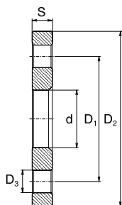
Volná příruba
