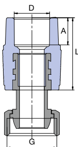
Eurokonus
