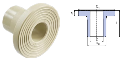
Lemový nákrůžek
