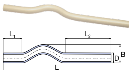
Křížení S 2,5 / PN 20 / SDR 6
