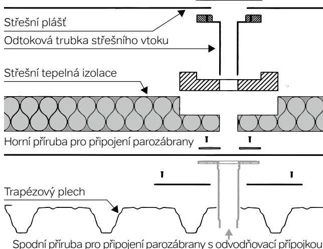
Instalace odvodňovací přípojky
